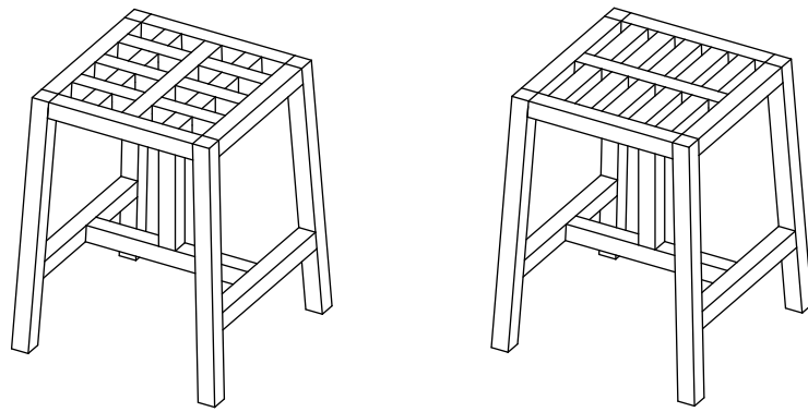
TWEEN STOOL
